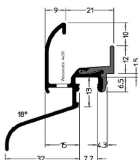
GUTMANN RSS KOCHER LOE 32 F TXL – BIJELA GUTMANN RSS KOCHER LOE 32 F TXL EV1 GUTMANN RSS KOCHER LOE 32 F TXL G214
