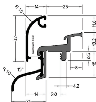
GUTMANN RSS DRAU 25/24 F-TI G214
