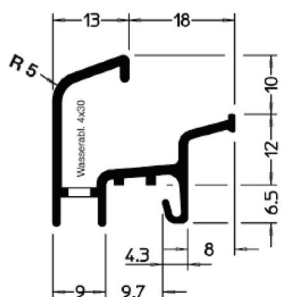
GUTMANN RSS DONAU 22F EV1 GUTMANN RSS DONAU 22F G214
