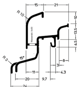
GUTMANN RSS ISAR 25/20F RAL9016
